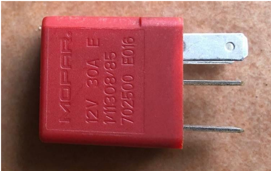
Relè nuovo:
